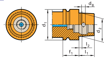
Form F DIN 69893 part 6
